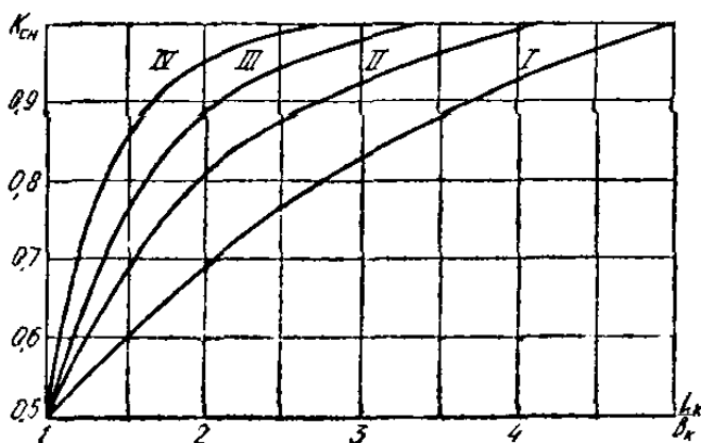
Рис. 6. Графики для определения коэффициента k_{сп}
