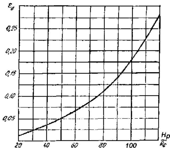
Рис. 3. График для определения \epsilon_0
