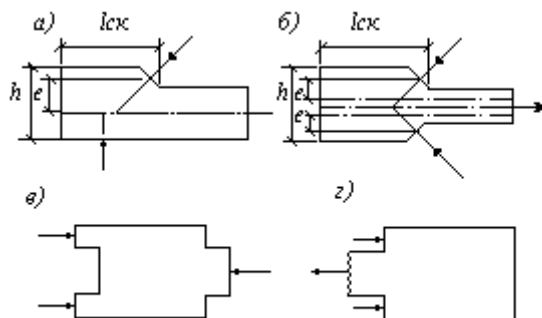
Рис. 5. Врезки в элементах соединений a – несимметричная; б – симметричная; в , г – схемы скальвания в соединениях
