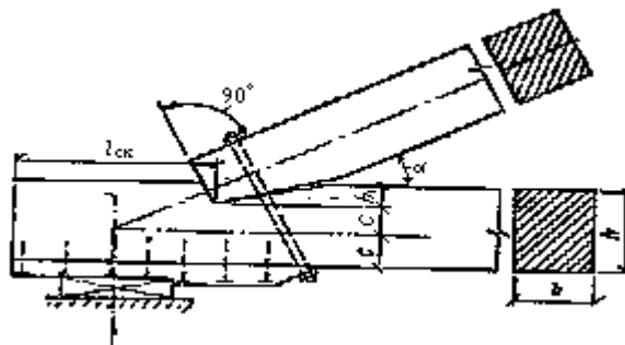
Рис. 7. Лобовая врубка с одним зубом
