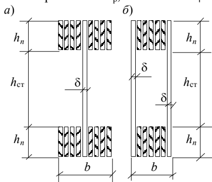
Рис. 4. Поперечные сечения клееных балок с плоской фанерной стенкой a – двутаврового сечения; b – коробчатого сечения
