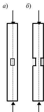
Рис. 1. Ослабление сжатых элементов а – не выходящие на кромку; б – выходящие на кромку
