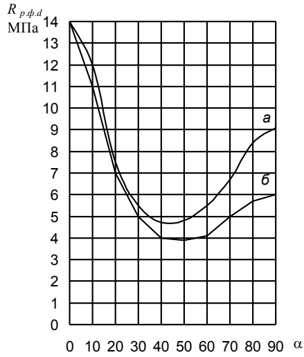
Рис. 17. Графики для определения расчетных сопротивлений при растяжении под углом к волокнам наружных слоев березовой фанеры марки ФСФ a – семислойной; б – пятислойной
