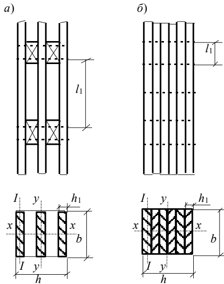
Рис. 2. Составные элементы а – с прокладками; б – без прокладок
