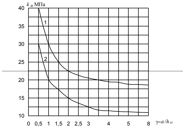
Рис. 17. Графики для определения расчетных сопротивлений при растяжении под углом к волокнам наружных слоев березовой фанеры марки ФСФ a – семислойной; б – пятислойной
