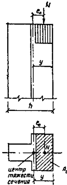
Рис. 5. Внецентренное сжатие
