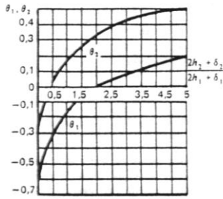
Черт.8. График для определения коэффициентов \theta_1 и \theta_2
