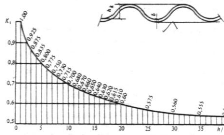
Черт.7. График для определения коэффициента K_1
