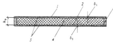
Черт.5. Поперечное сечение бескаркасной панели с обрамлением
