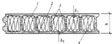
Черт.4. Поперечное сечение экструзионной панели
